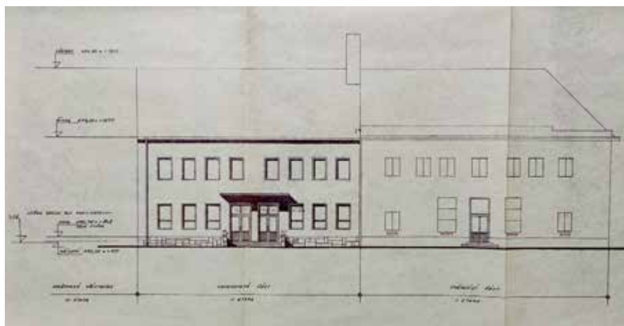
Obr. 2 Výřez stavebního plánu z roku 1970, čelní fasáda (Stavební úřad Vyšší Brod)
