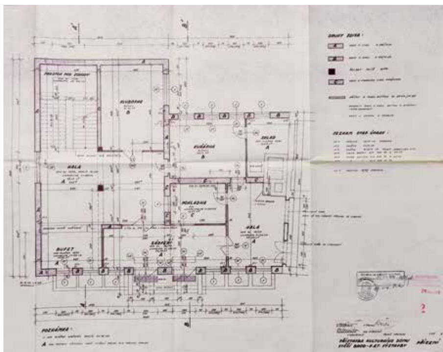
Obr. 3 Stavební plán z roku 1970, půdorys přízemí (Stavební úřad Vyšší Brod)
